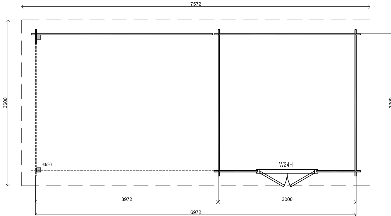
Plattegrond / Plan
