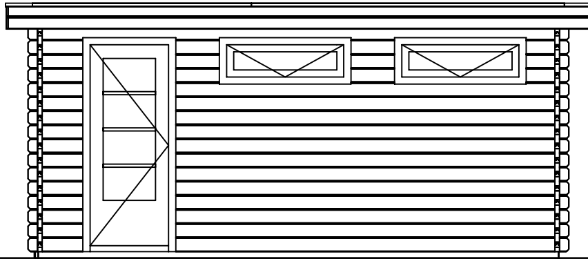
Vooraanzicht / Front view / Vorderansicht 5600
